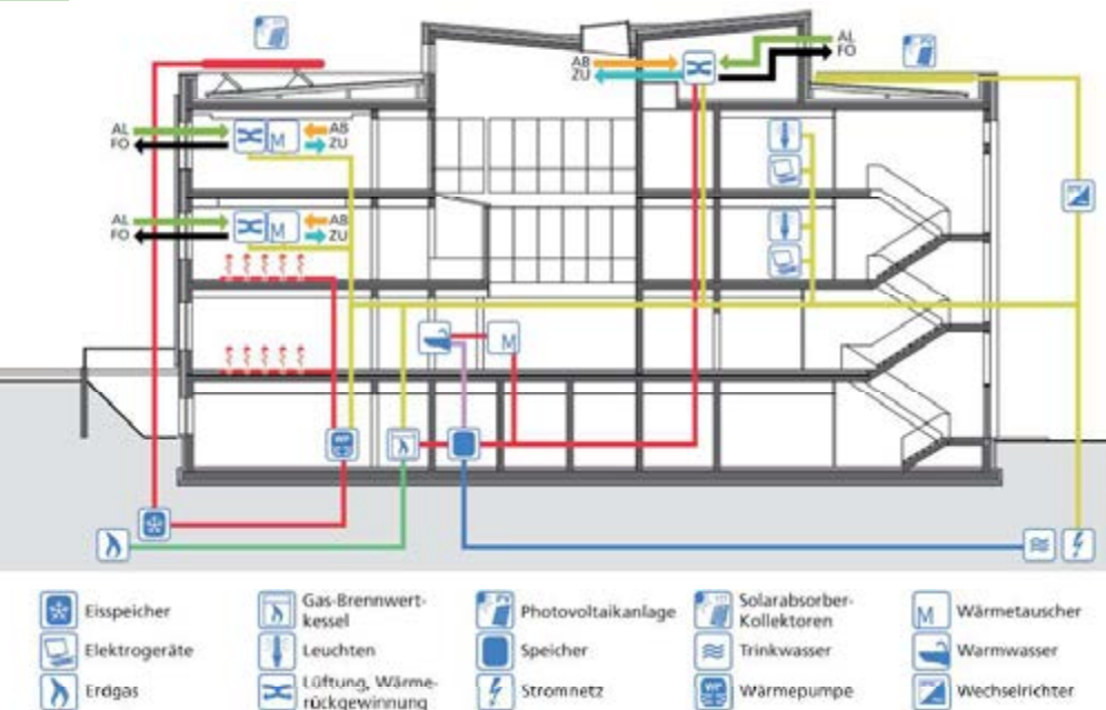
Anlagentechnik: Längsschnitt durch das Gebäude und Konzeption der Haustechnik - Grafik: Fraunhofer IBP
