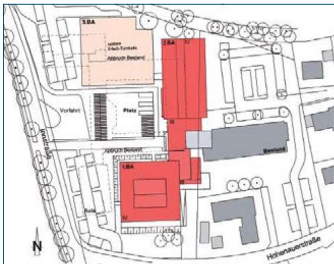
Lageplan der Gesamtanlage des neuen Berufsschulzentrums Mühlendorf - Plan: ARGE Schmuck-Anghuber Architekten
